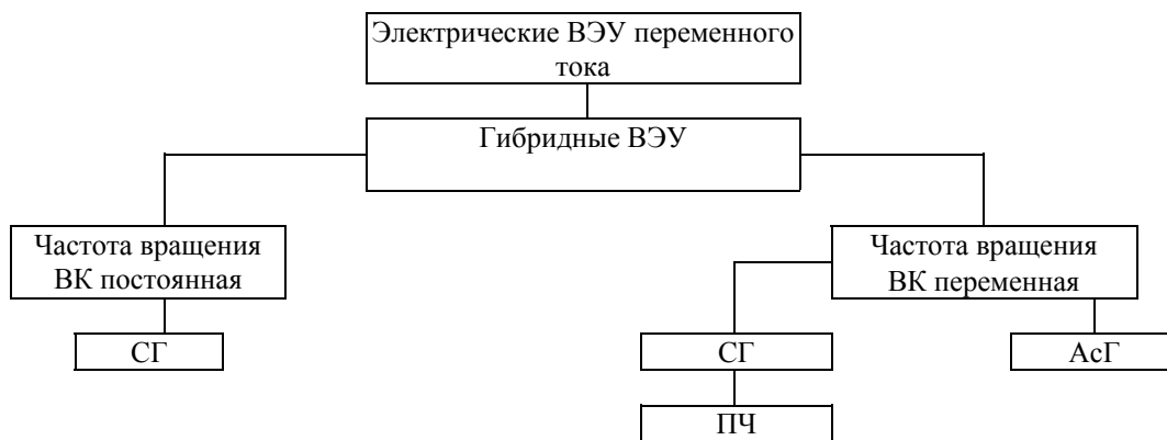
Рисунок 2 — Структурная схема автономных ВЭУ
